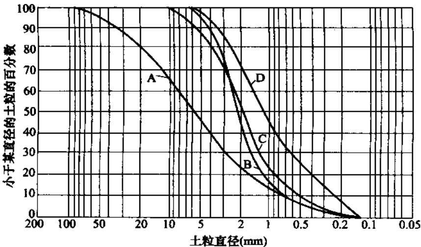
图 1 判别冲积层可灌性的颗粒级配曲线
