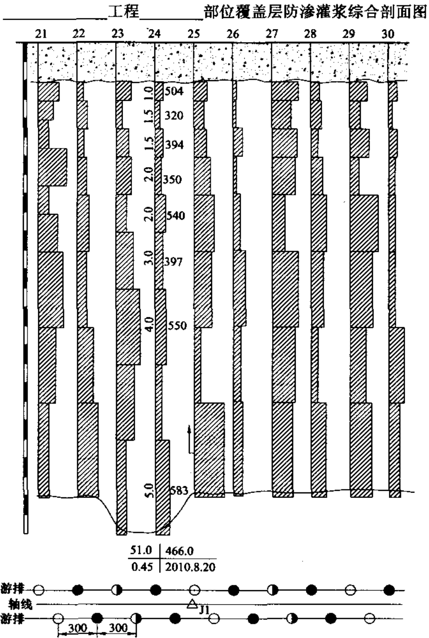
图 B.0.1 覆盖层防渗帷幕灌浆综合剖面图（孔口封闭）
